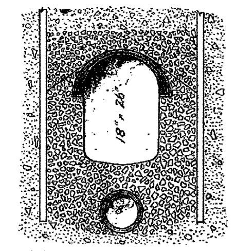
CONCRETE ENCASUREMENT DETAIL N.T.S.
