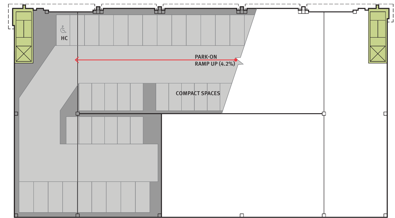
ROOF PLAN //
