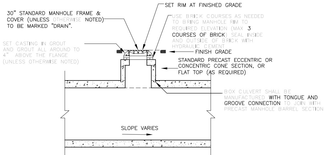
LONGITUDINAL SECTION
