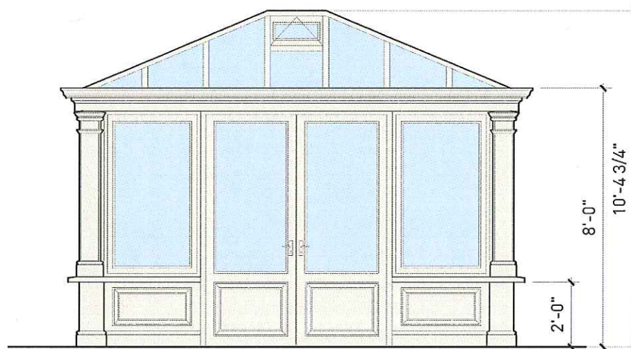
END ELEVATION
