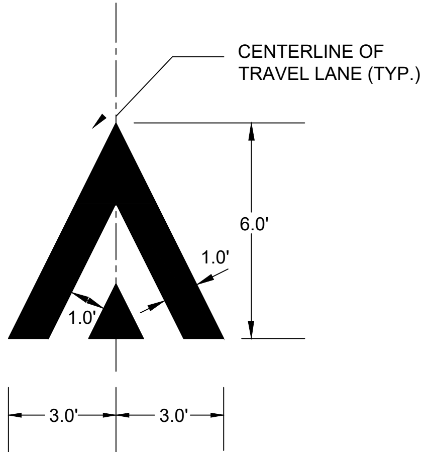
RAMP MARKING DETAIL SCALE: N.T.S.
